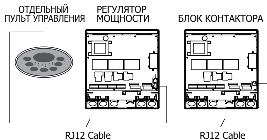
Рис.6 Установка отдельного пульта управления с регулятором мощности и блоком контактора
