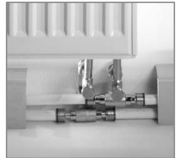
Подключение радиатора с использованием двойного тройника при плитусной проводке
