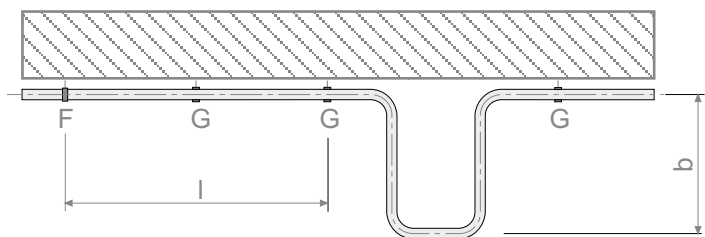
Пример оборудования компенсатора на прямолинейном участке трубопровода
