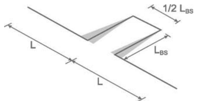
Компенсатор теплового удлинения
