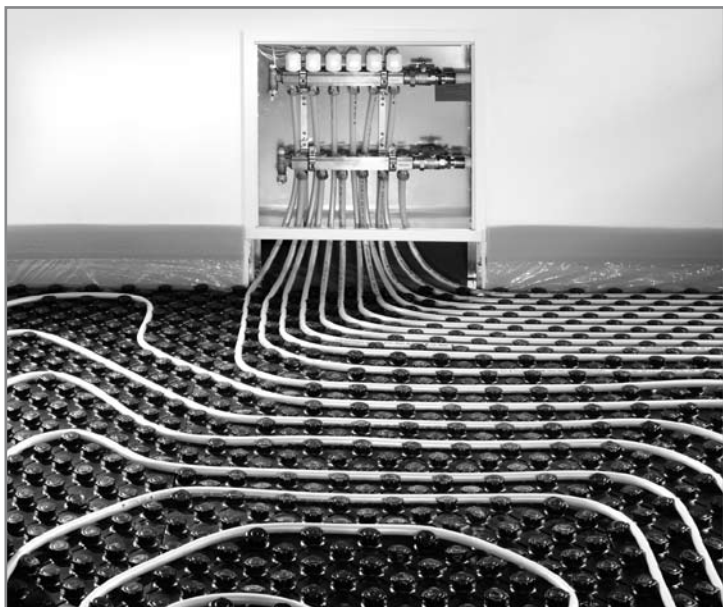
Укладка труб с применением полистирольных плит TECeFlex
