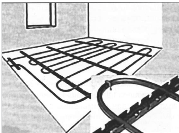
Укладка труб с применением рулонной полистирольной изоляции и направляющих планок для укладки труб
