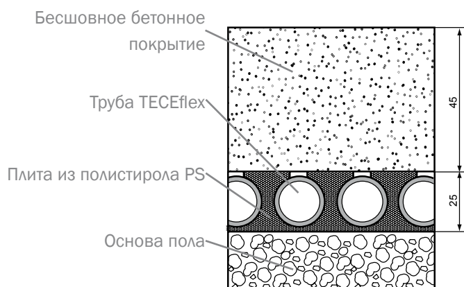
Схема укладки труб с применением полистирольных плит TECeFlex
