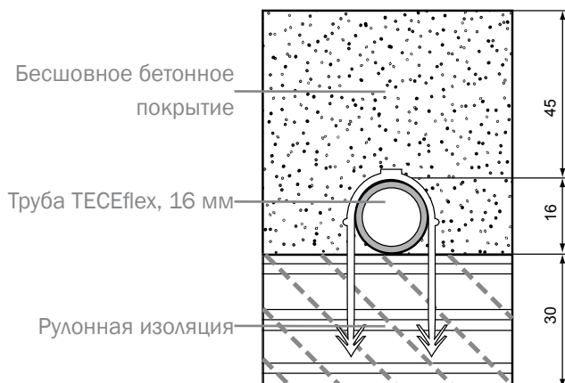
Схема укладки труб с применением полистирольной рулонной изоляции и якорных клипс
