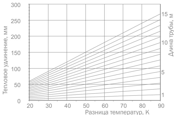
Температурное удлинение для труб РЕ-Хс и РЕ-MDXc TECeFlex
