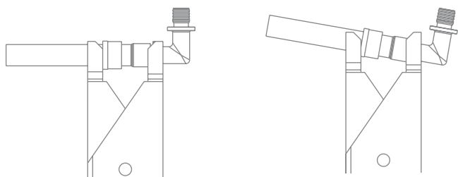
Прессование: слева — правильно; справа — неправильно
