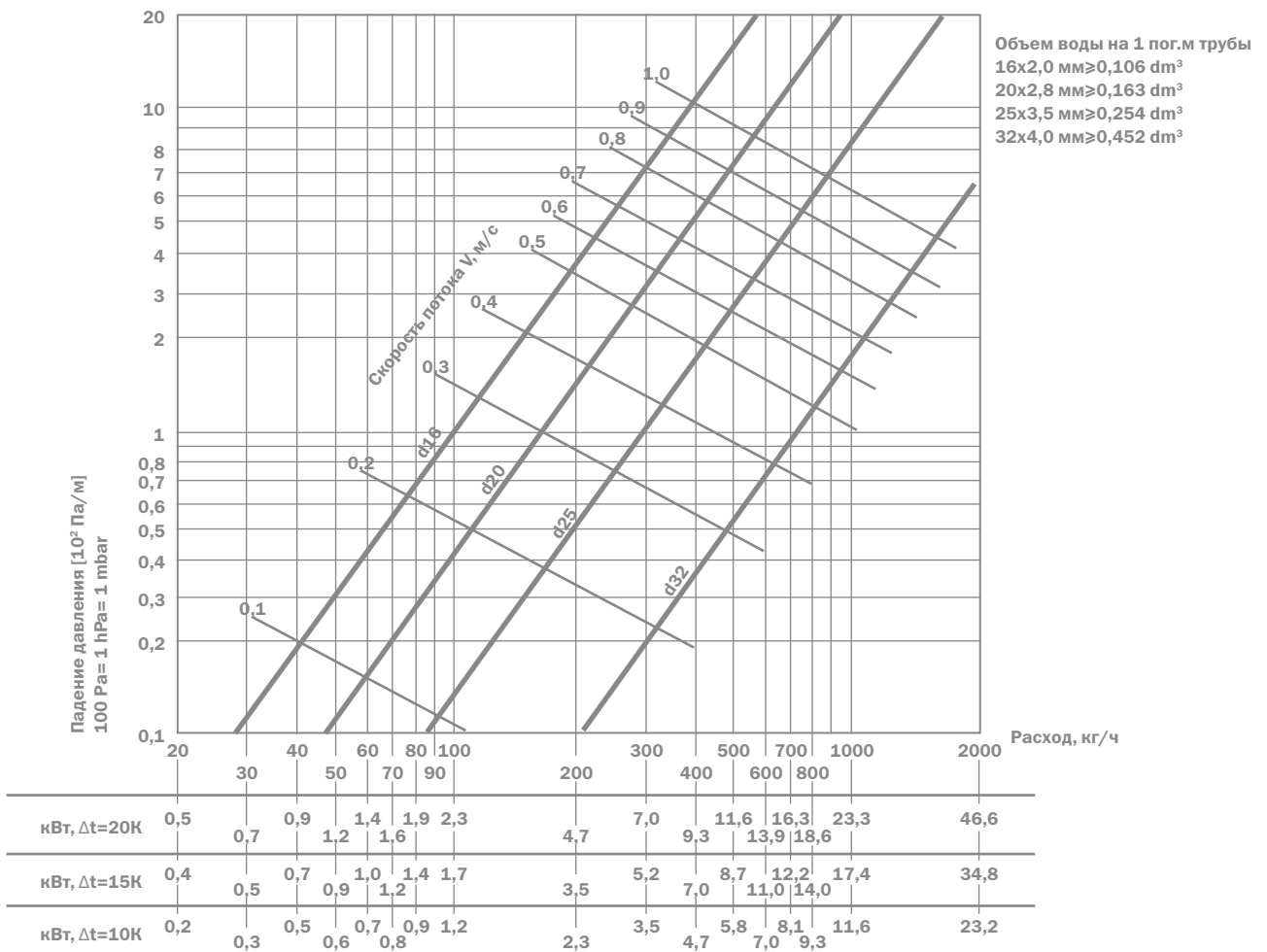
Диаграмма падения давления для универсальных многослойных труб в системах отопления
