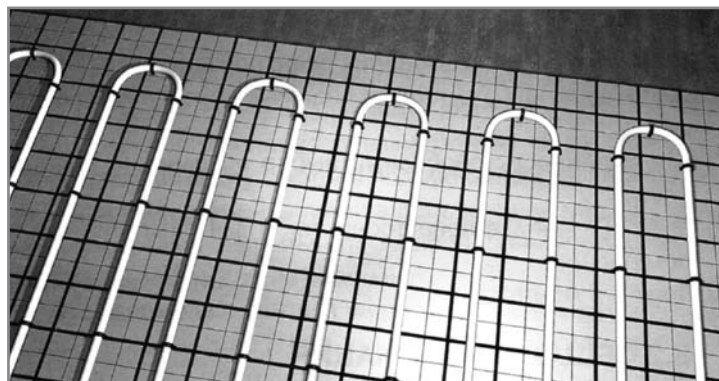
Укладка труб с применением рулонной полистирольной изоляции и якорных клипс TECeFlex
