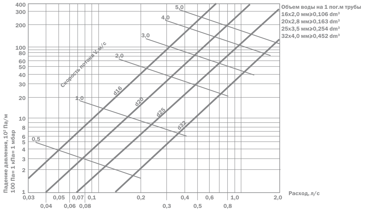
Диаграмма падения давления для универсальных многослойных труб в системах отопления
