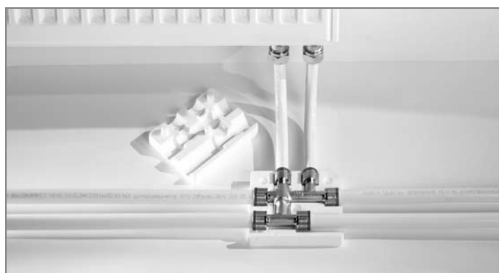
Подключение радиатора с использованием двойного тройника
