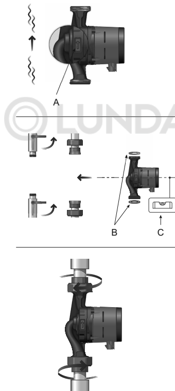
Рис. 3 Монтаж насоса ALPHA3
