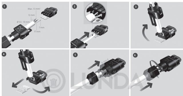
Рис. 9 Установка электророзъема
