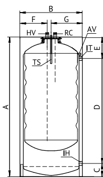
Напольный F350
