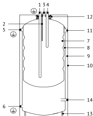
Напольный F160-300
