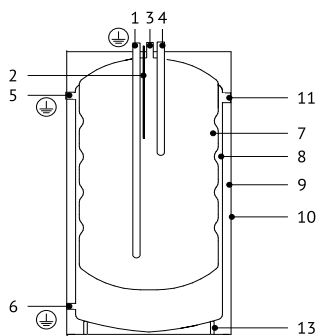
Напольный F100
