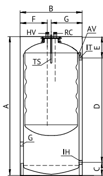
Напольный F160-300
