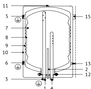
Настенный W100-230
