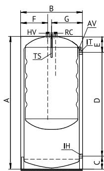
Напольный F100
