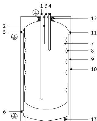
Напольный F350
