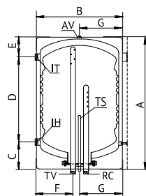
Настенный W100-230
