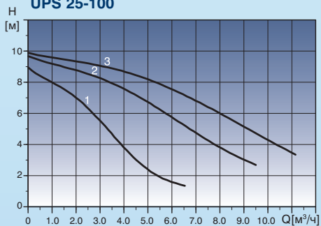
UPS 25-100
