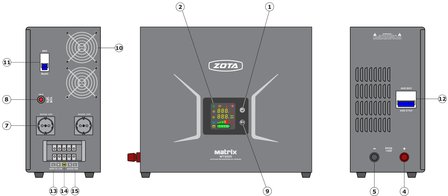
Рис.2 Элементы управления инвертора Matrix-WT2100....Matrix-WT5000.
