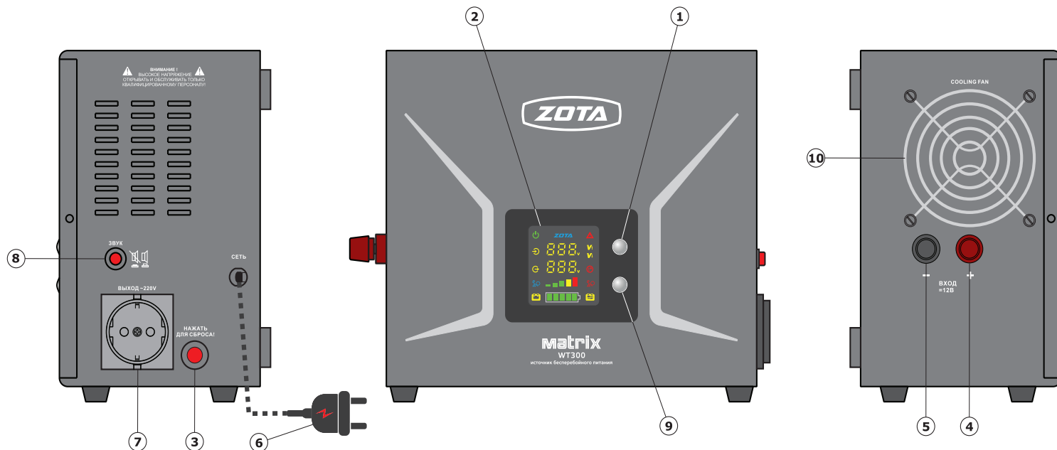
Рис.1 Элементы управления инвертора Matrix-WT300....Matrix-WT1800.
